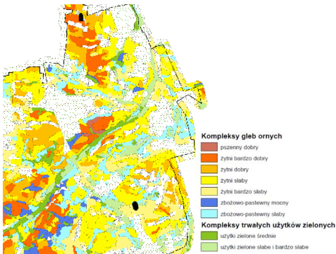
Rysunek 9. Fragment mapy glebowo-rolniczej 1:25 000 Kompleksy gleb (źródło: PIG, PUWG 1992)
