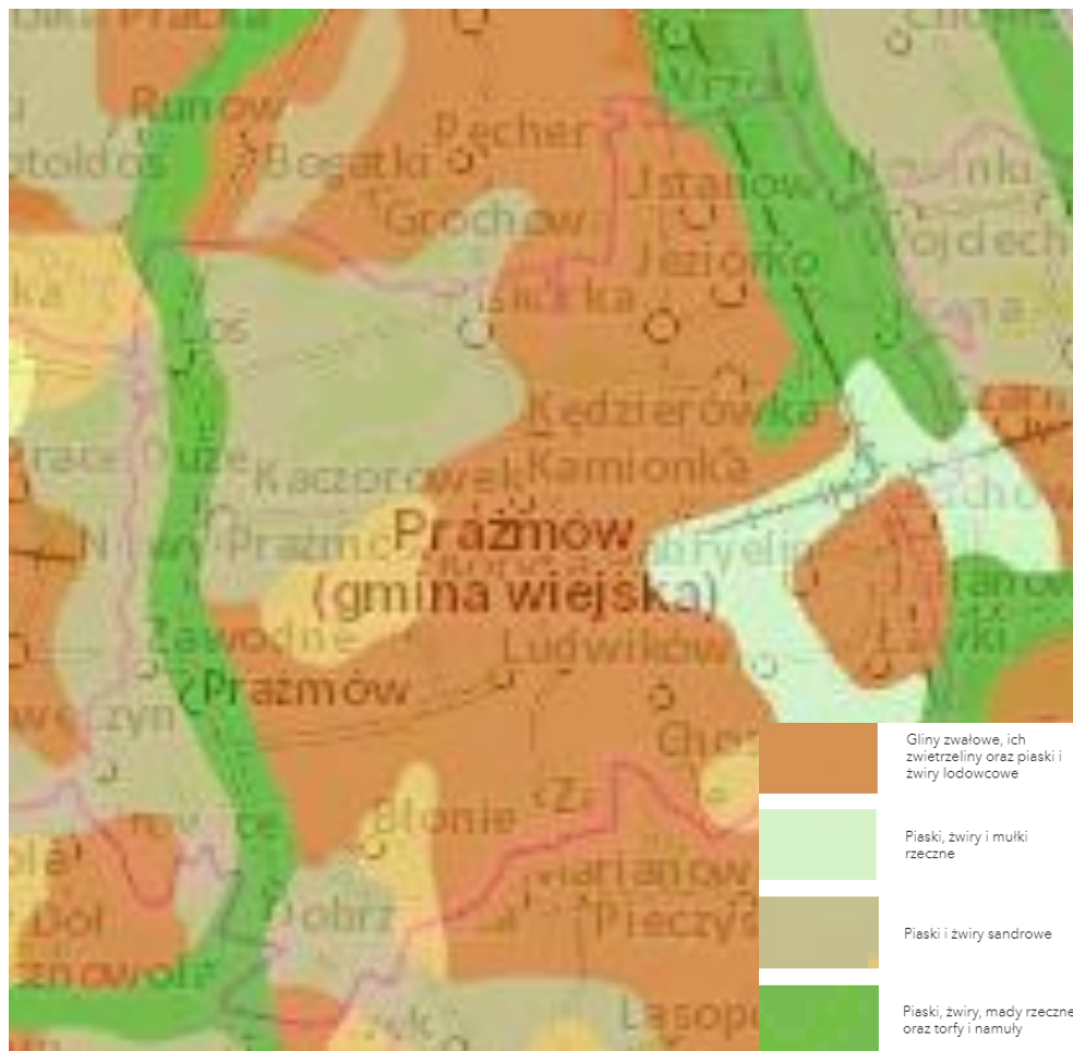
Rysunek 5. Fragment mapy geologicznej 1:500 000 (źródło: http://bazagis.pgi.gov.pl )
