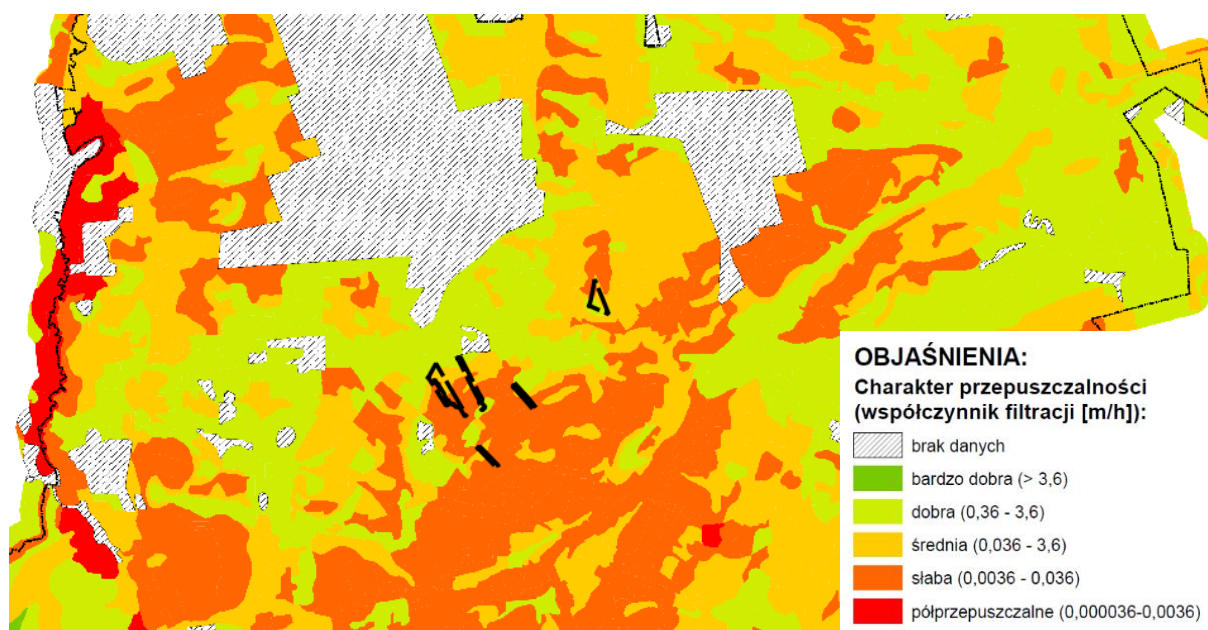
Rysunek 13. Fragment mapy glebowo-rolniczej 1:25 000 Charakter przepuszczalności (źródło: PIG, PUWG 1992)
