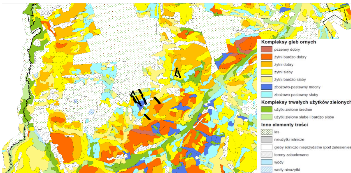
Rysunek 10. Fragment mapy glebowo-rolniczej 1:25 000 Kompleksy gleb (źródło: PIG, PUWG 1992)
