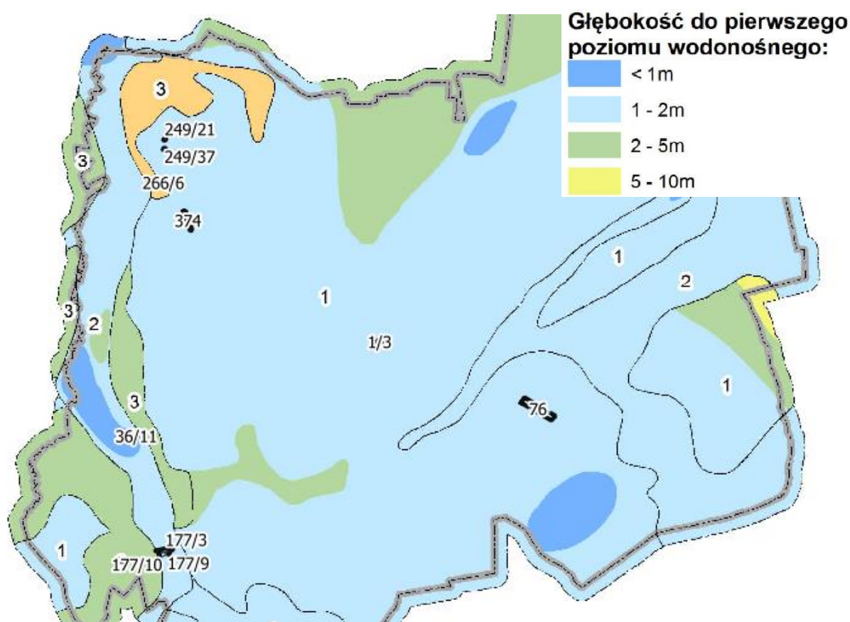
Rysunek 13. Fragment mapy głębokości pierwszego poziomu wodonośnego
