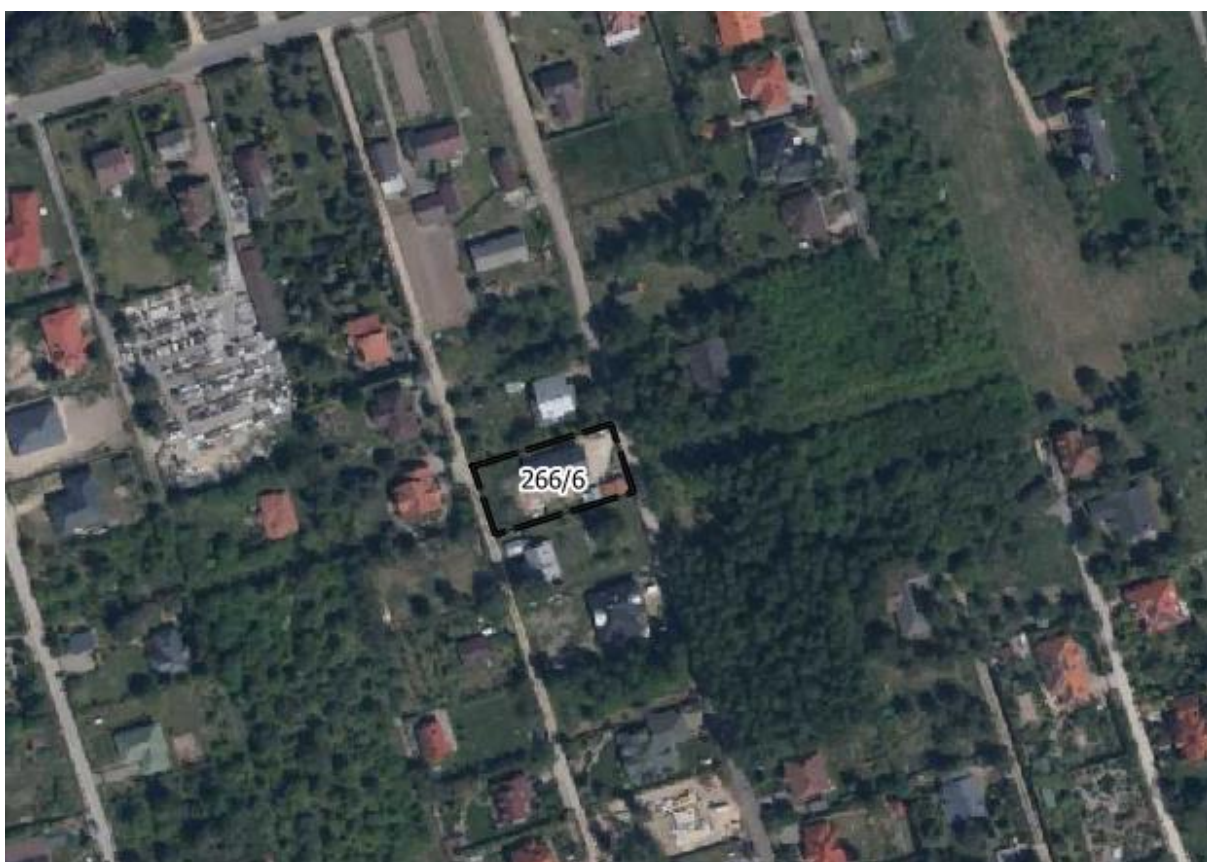
Rysunek 4. Ortofotomapa analizowanego obszaru w Łosiu ( www.geoportal.gov.pl )
