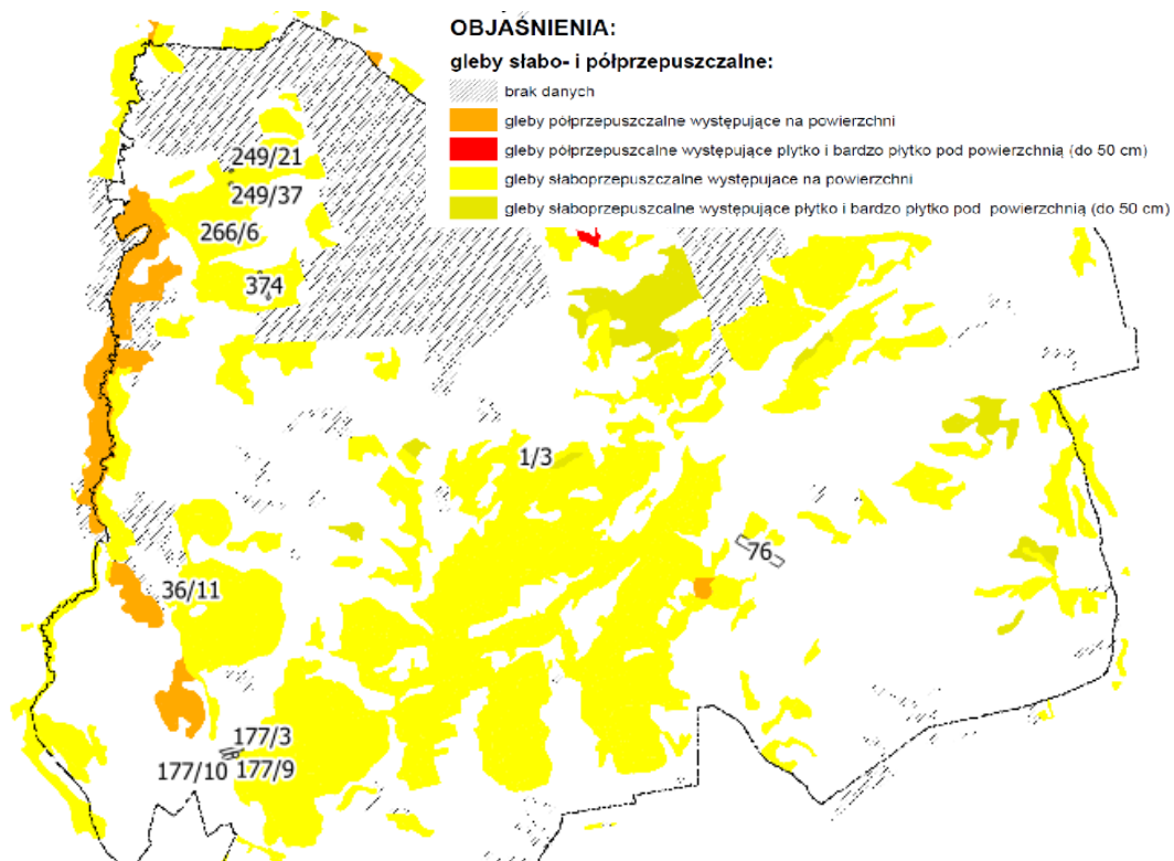
Rysunek 18. Fragment mapy glebowo-rolniczej 1:25 000 Gleby słabo- i półprzepuszczalne (źródło: PIG, PUWG 1992)
