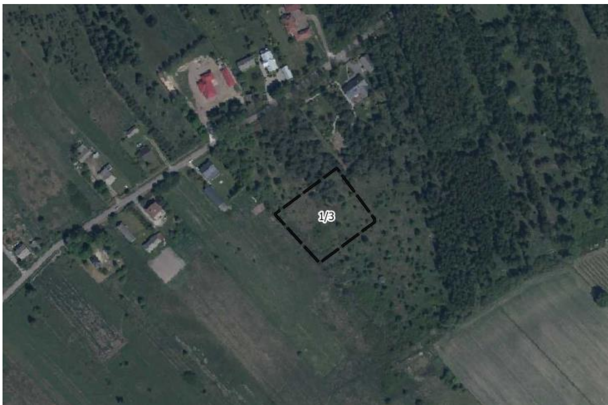
Rysunek 9. Ortofotomapa analizowanego obszaru w Ludwikowie ( www.geoportal.gov.pl )
