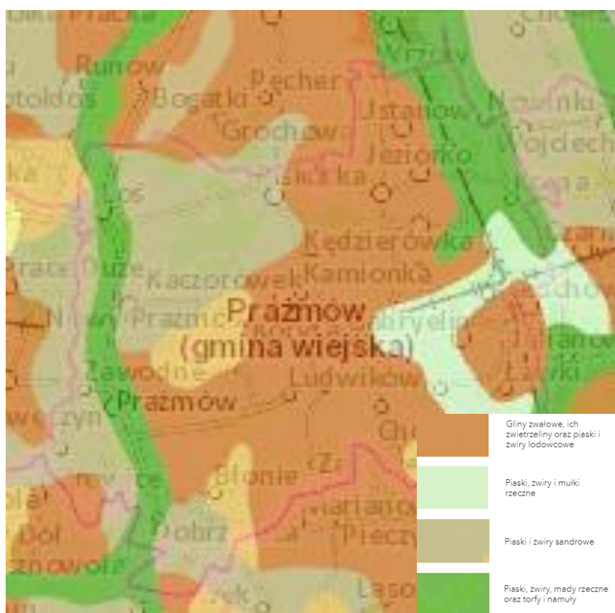
Rysunek 12. Fragment mapy geologicznej 1:500 000 (źródło: http://bazagis.pgi.gov.pl )
