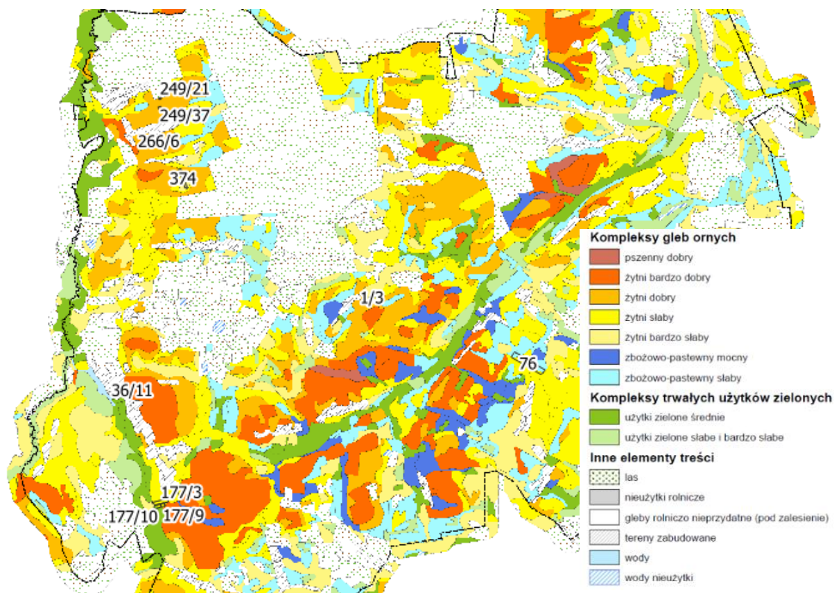
Rysunek 16. Fragment mapy glebowo-rolniczej 1:25 000 Kompleksy gleb (źródło: PIG, PUWG 1992)
