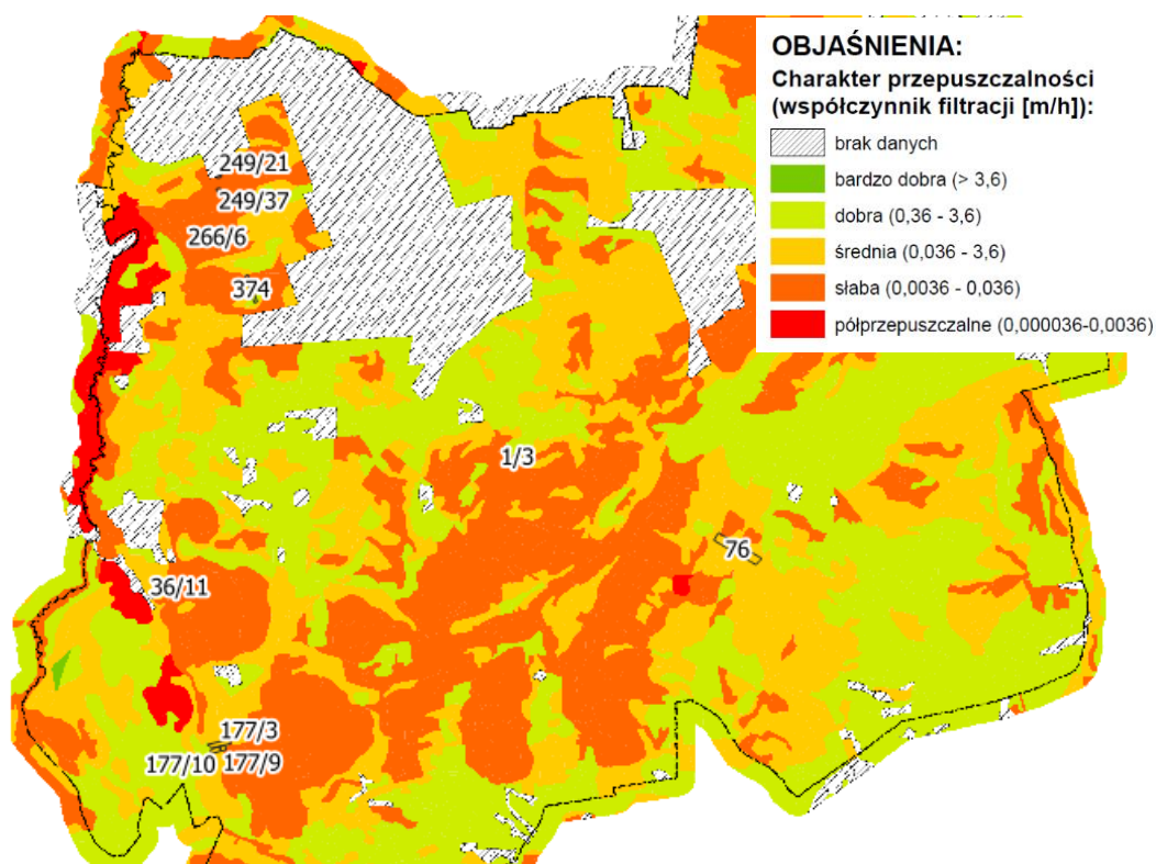
Rysunek 19. Fragment mapy glebowo-rolniczej 1:25 000 Charakter przepuszczalności (źródło: PIG, PUWG 1992)
