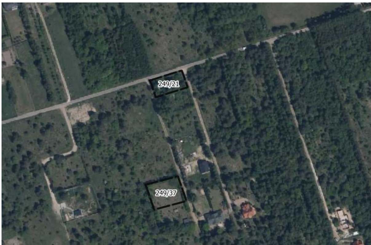
Rysunek 3. Ortofotomapa analizowanych obszarów w Łosiu ( www.geoportal.gov.pl )
