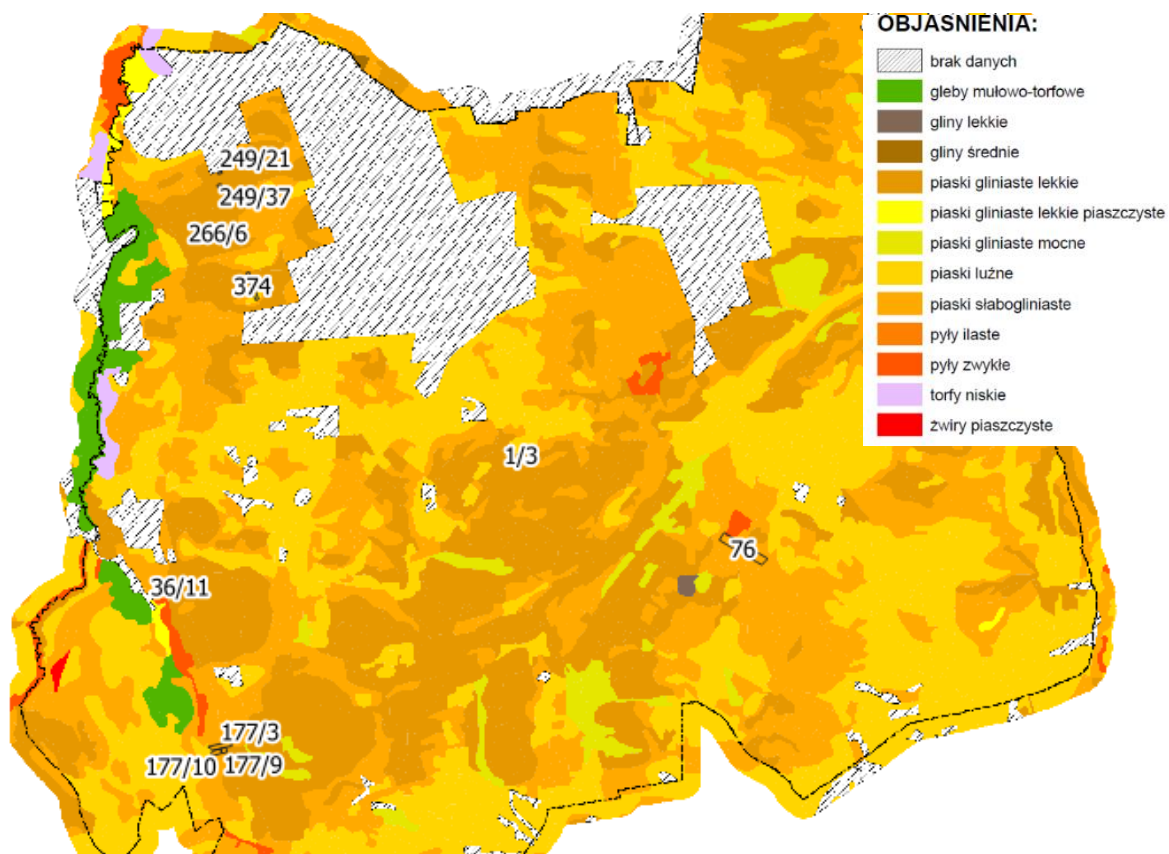
Rysunek 17. Fragment mapy glebowo-rolniczej 1:25 000 Rodzaje i gatunki gleb (źródło: PIG, PUWG 1992)
