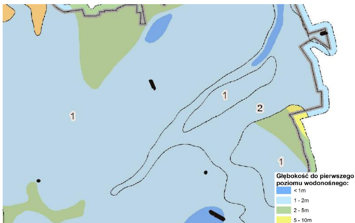
Rysunek 11. Fragment mapy głębokości pierwszego poziomu wodonośnego
