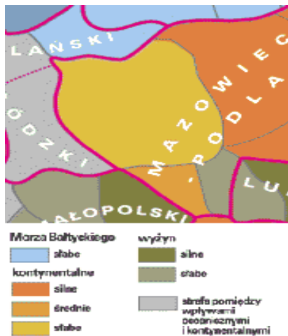
Rysunek 13. Podział klimatyczny R. Guminskiego
