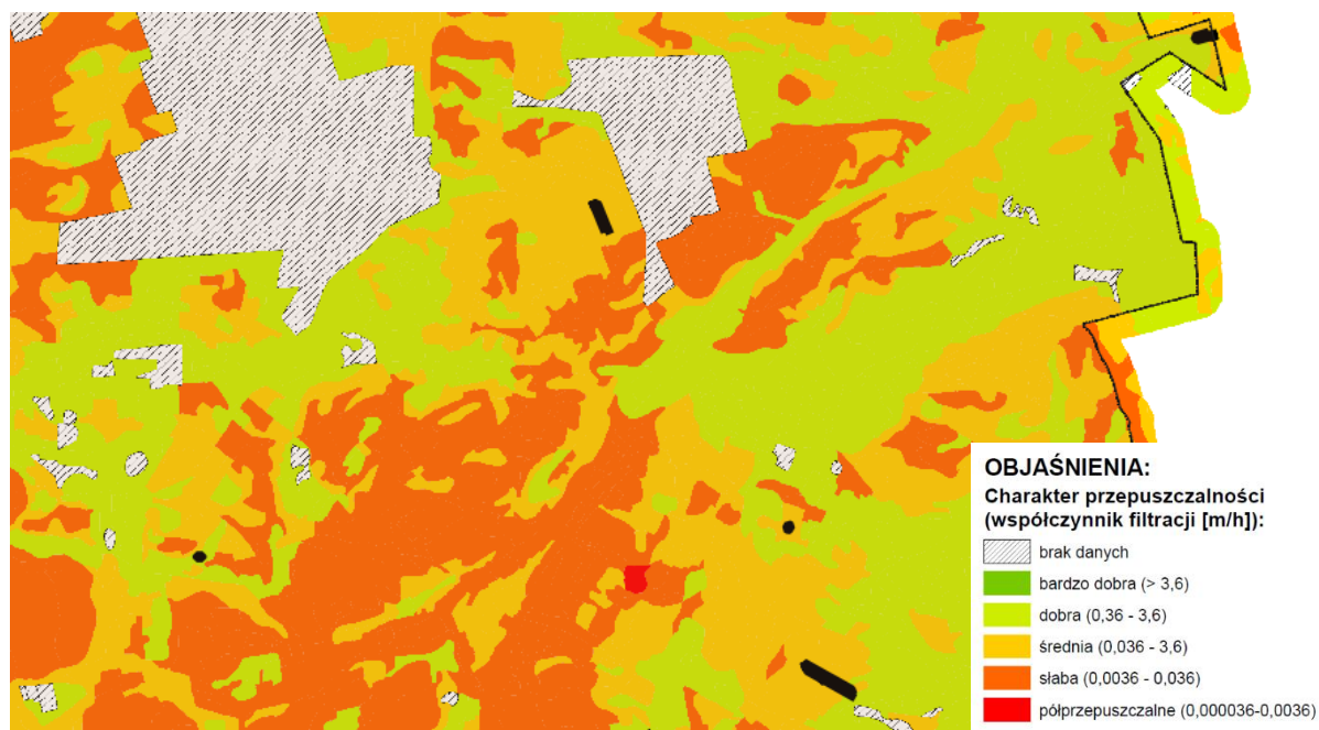
Rysunek 17. Fragment mapy glebowo-rolniczej 1:25 000 Charakter przepuszczalności (źródło: PIG, PUWG 1992)
