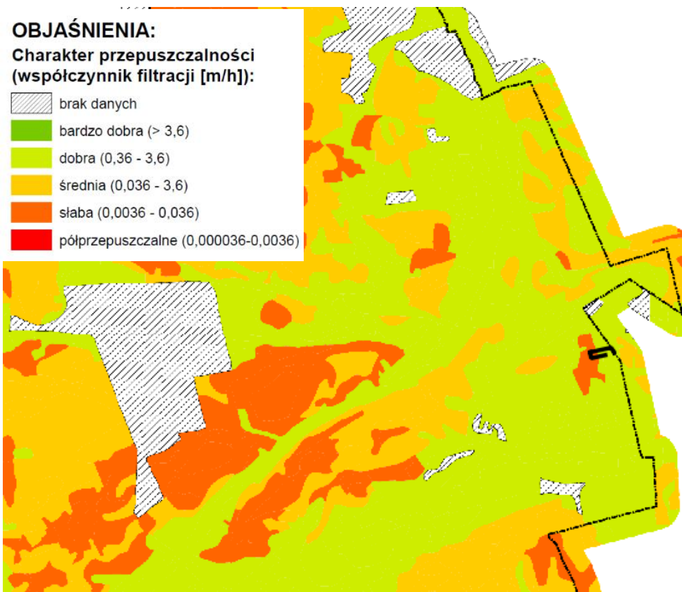
Rysunek 13. Fragment mapy glebowo-rolniczej 1:25 000 Charakter przepuszczalności (źródło: PIG, PUWG 1992)
