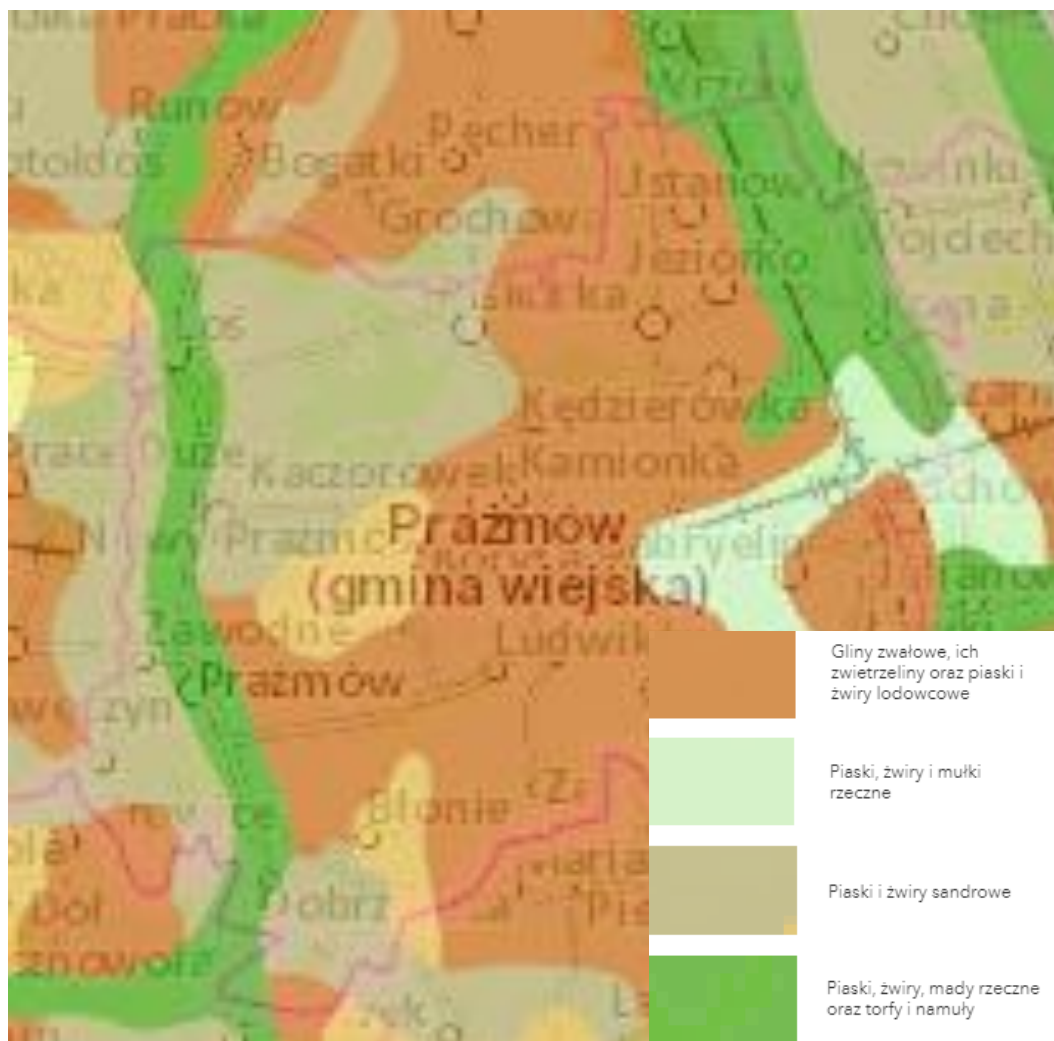
Rysunek 6. Fragment mapy geologicznej 1:500 000 (źródło: http://bazagis.pgi.gov.pl )
