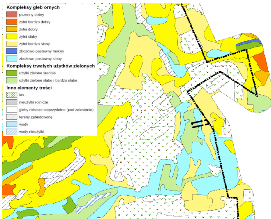
Rysunek 10. Fragment mapy glebowo-rolniczej 1:25 000 Kompleksy gleb (źródło: PIG, PUWG 1992)
