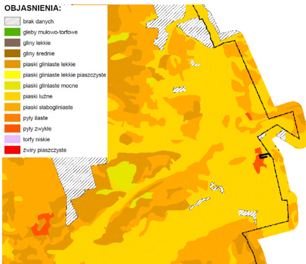
Rysunek 11. Fragment mapy glebowo-rolniczej 1:25 000 Rodzaje i gatunki gleb (źródło: PIG, PUWG 1992)
