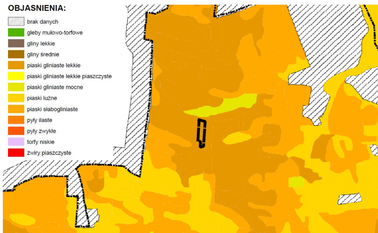
Rysunek 9. Fragment mapy glebowo-rolniczej 1:25 000 Rodzaje i gatunki gleb (źródło: PIG, PUWG 1992)
