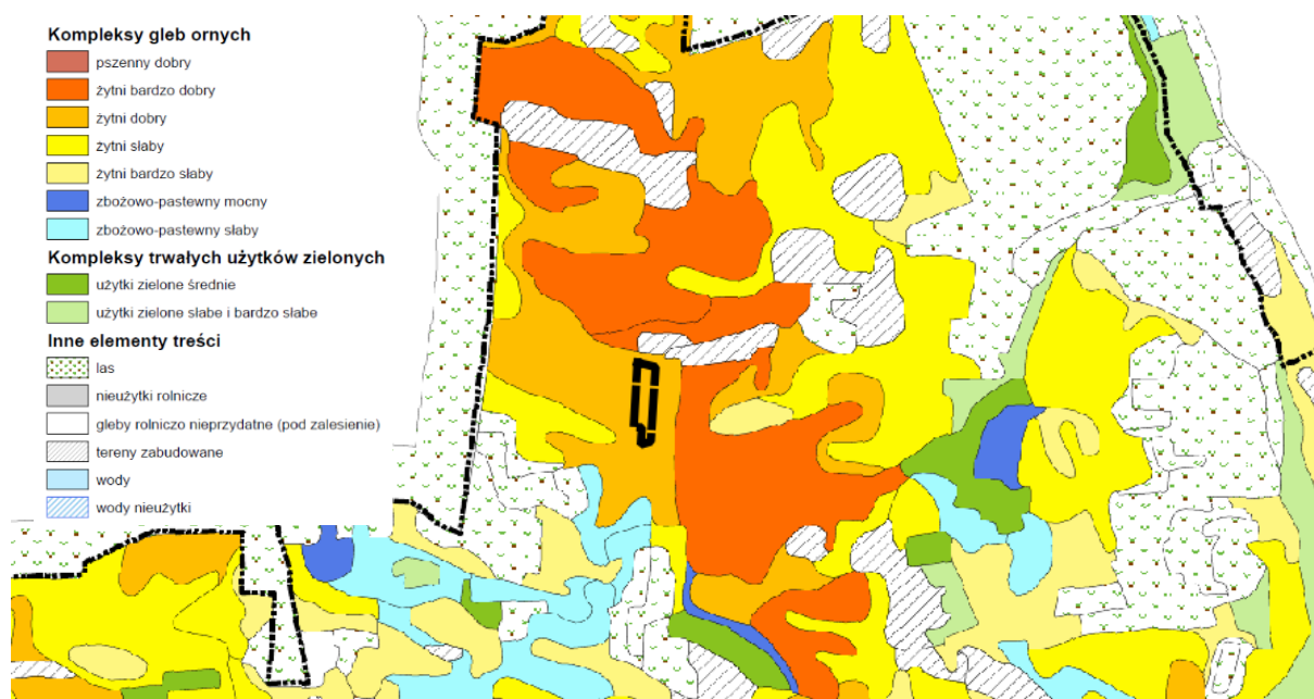
Rysunek 8. Fragment mapy glebowo-rolniczej 1:25 000 Kompleksy gleb (źródło: PIG, PUWG 1992)
