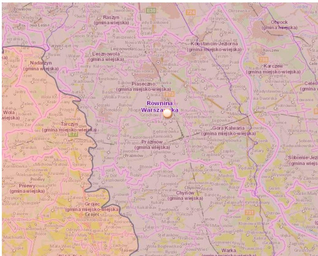
Rysunek 3. Położenie terenu opracowania na tle regionów fizycznogeograficznych wprowadzonego przez J. Konradzkiego, (Geografia regionalna Polski, Warszawa 2002)
