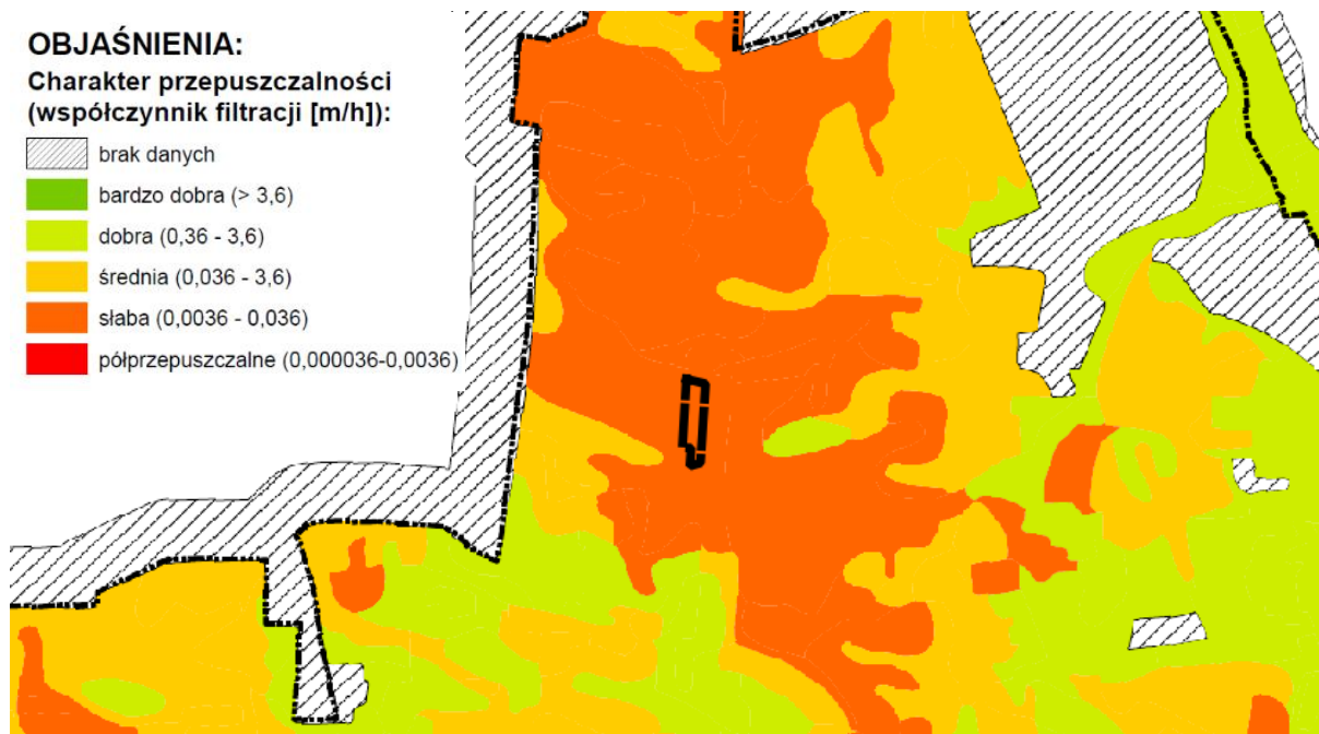
Rysunek 11. Fragment mapy glebowo-rolniczej 1:25 000 Charakter przepuszczalności (źródło: PIG, PUWG 1992)
