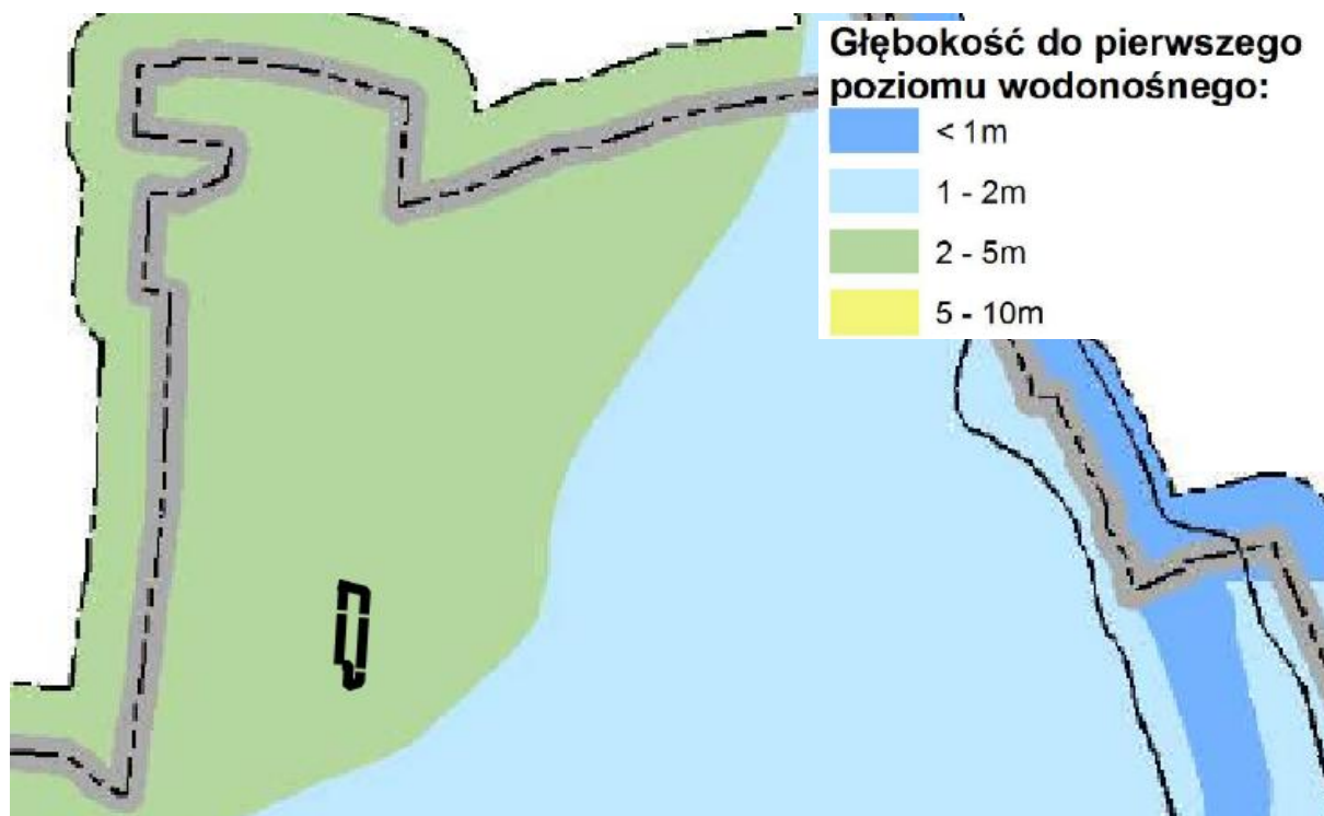
Rysunek 5. Fragment mapy głębokości pierwszego poziomu wodonośnego
