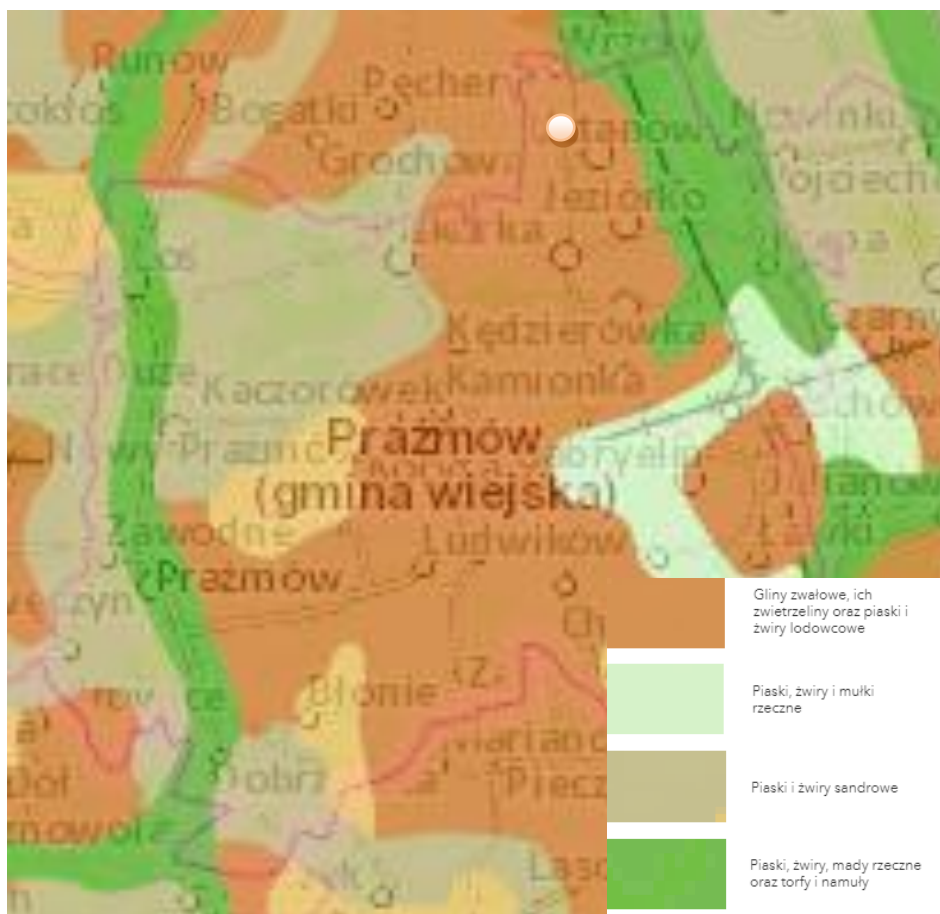
Rysunek 4. Fragment mapy geologicznej 1:500 000 (źródło: http://bazagis.pgi.gov.pl )
