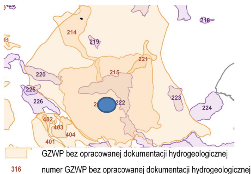
Rysunek 6. Lokalizacja terenu na tle GZWP
