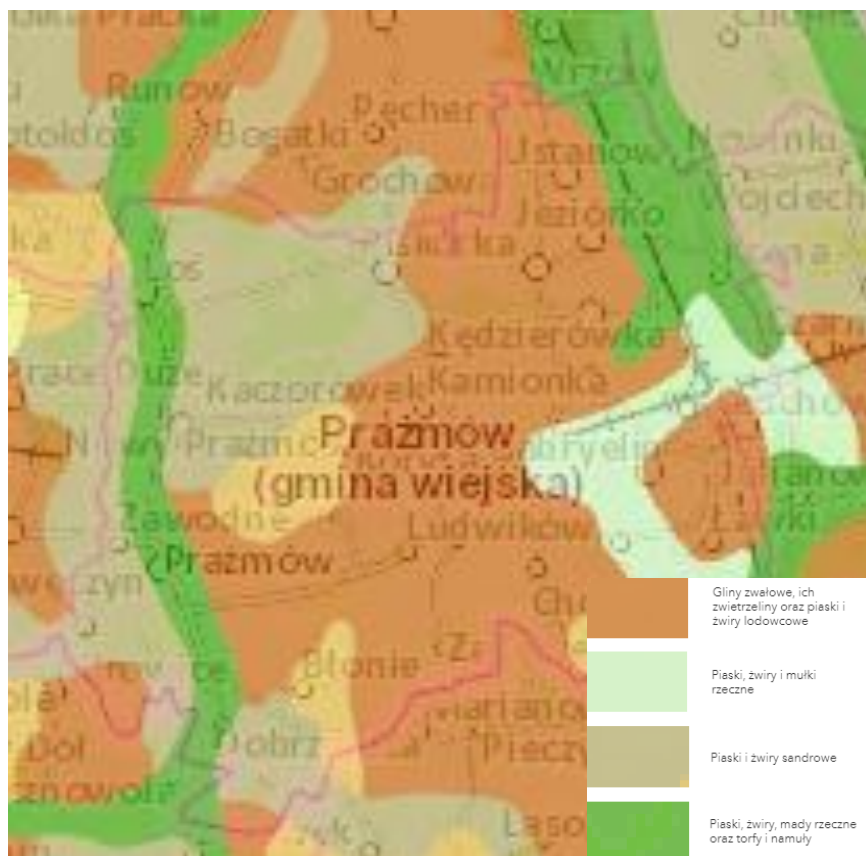
Rysunek 6. Fragment mapy geologicznej 1:500 000 (źródło: http://bazagis.pgi.gov.pl )
